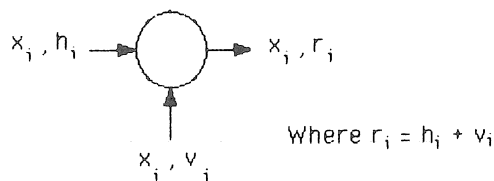
(d) Adder
